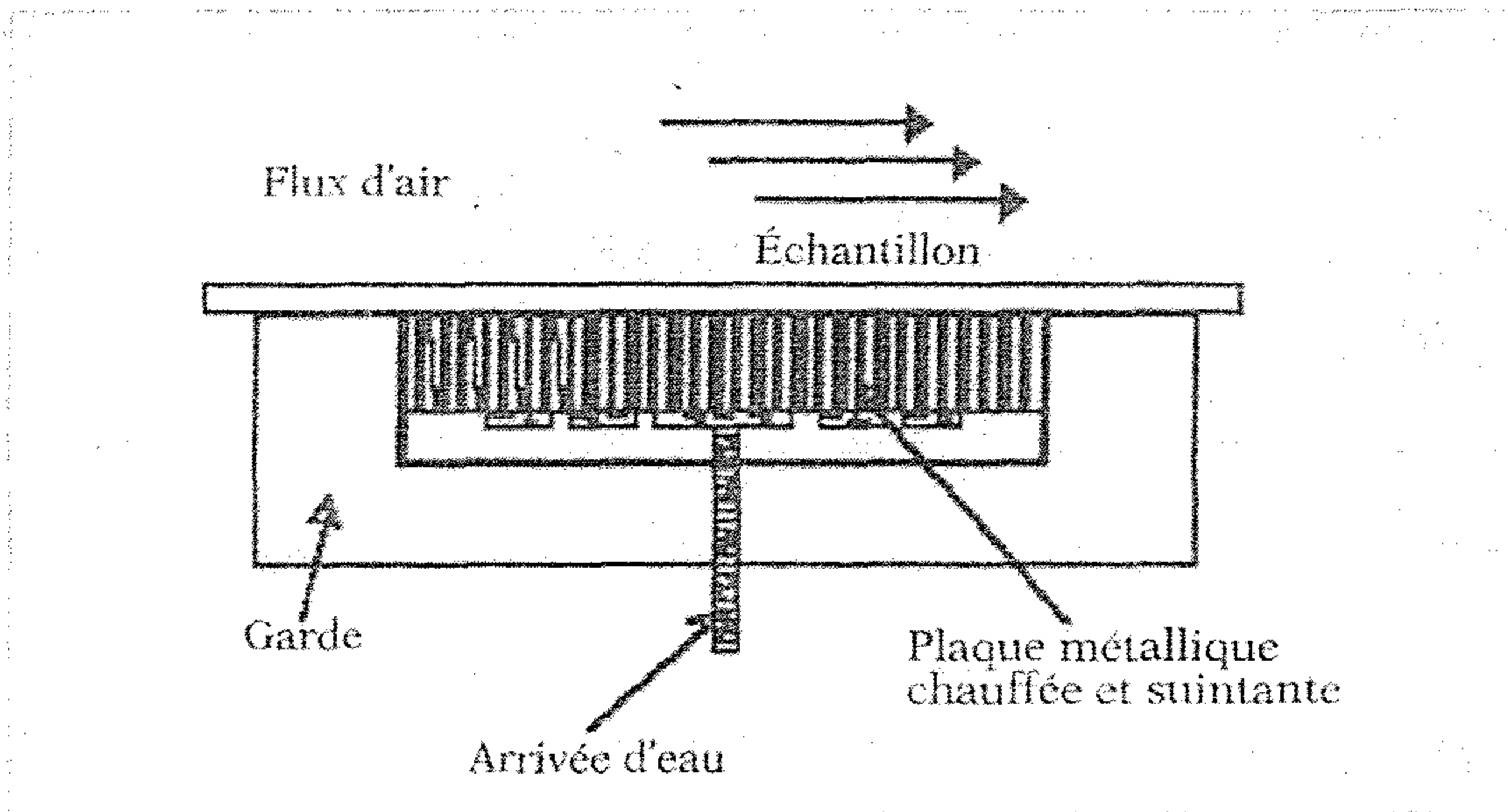
Figure 1 - La résistance évaporative est définie par : R_e = (P_{skin} - P_{air})/H_e La résistance thermique est définie par : R_c = (T_{skin} - T_{air})/H_c Skin model (iso 11092)
